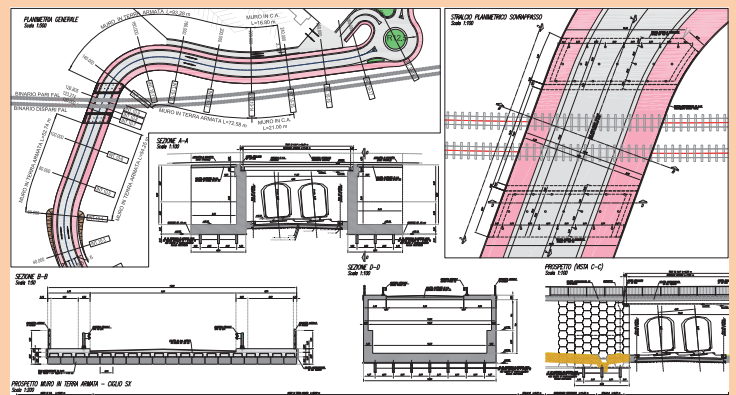
Dettagli sovrapasso ferroviario
